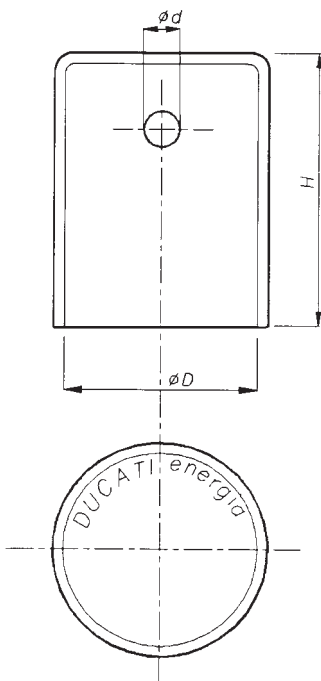
Fig. 9 Cappello. Fig. 9 Protective cap.
